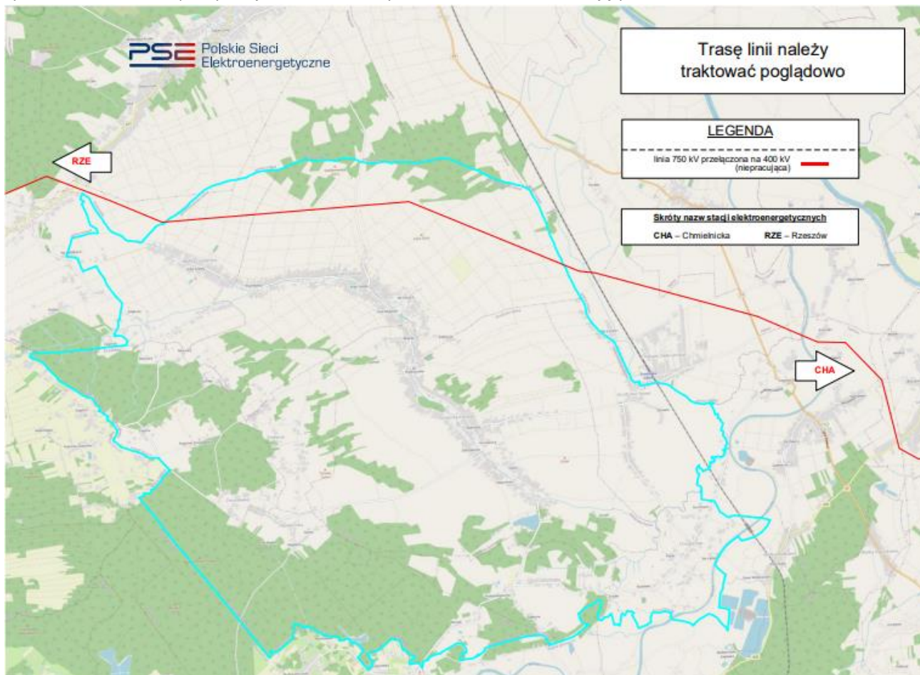
Rysunek 3. Schemat sieci przesyłowej na obszarze Gminy Grodzisko Dolne – stan istniejący.
